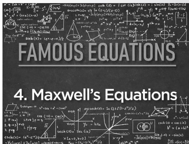
Maxwellove rovnice
